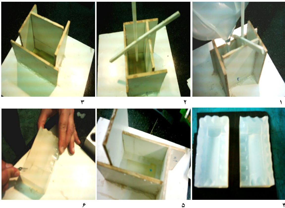
شکل (۸): مراحل گوناگون ساخت قالب RTV (از راست به چپ و از بالا به پایین)
