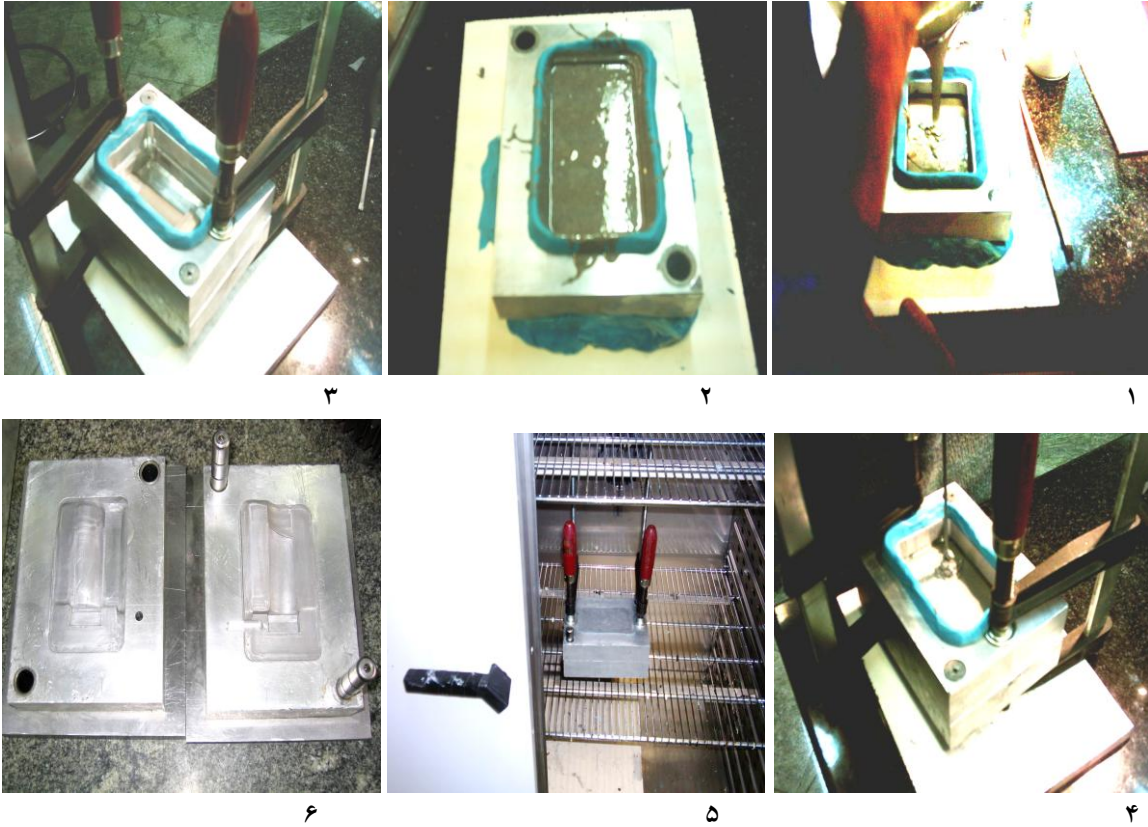
شکل (۷): مراحل گوناگون ساخت قالب اپوکسی (از راست به چپ و از بالا به پایین)
